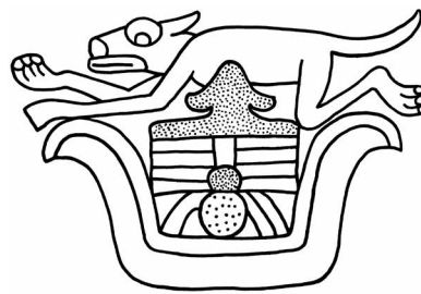
Figura 7. Recipientes de nacimiento y sacrificio representados en el Códice Borgia: (a) escena de probable bautismo con infante demoníaco en recipiente de cráneo; detalle de la p. 31 del Códice Borgia; (b) Quetzalcóatl y cinco Tezcatlipocas que nacen de cuchillos de pedernal sobre personaje acucillado; detalle de la p. 32 del Códice Borgia—nótese la cadera en forma de recipiente de cráneo que contiene cuchillos de sacrificio; (c) Quetzalcóatl emergiendo de la parte media de diosa; detalle de la p. 32 del Códice Borgia—comparar el perfil del orificio con los tazones en d-e ; (d) recipiente de ofrendas que contiene animal sacrificado; detalle de la p. 22 del Códice Fejérváry-Mayer; (e) tazón que contiene corazón y sangre, sostenido por la diosa Chalchiuhtlicue; detalle de la p. 20 del Códice Borgia.
