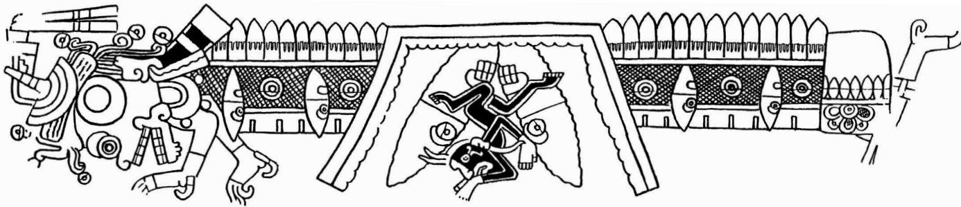
Figura 7. Recipientes de nacimiento y sacrificio representados en el Códice Borgia: (a) escena de probable bautismo con infante demoníaco en recipiente de cráneo; detalle de la p. 31 del Códice Borgia; (b) Quetzalcóatl y cinco Tezcatlipocas que nacen de cuchillos de pedernal sobre personaje acucillado; detalle de la p. 32 del Códice Borgia—nótese la cadera en forma de recipiente de cráneo que contiene cuchillos de sacrificio; (c) Quetzalcóatl emergiendo de la parte media de diosa; detalle de la p. 32 del Códice Borgia—comparar el perfil del orificio con los tazones en d-e ; (d) recipiente de ofrendas que contiene animal sacrificado; detalle de la p. 22 del Códice Fejérváry-Mayer; (e) tazón que contiene corazón y sangre, sostenido por la diosa Chalchiuhtlicue; detalle de la p. 20 del Códice Borgia.
