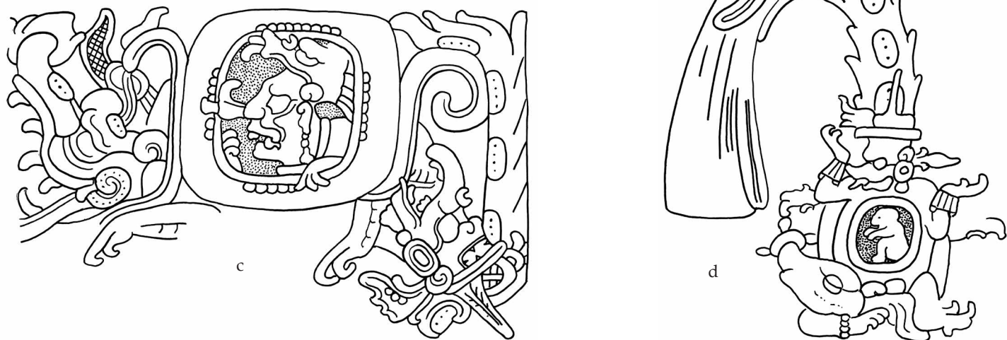
Figura 18. Representación maya del período Clásico de seres con características de saurio y tazones marcados con el signo k'in en el área de los genitales: (a) Cocodrilo-Venado Estrellado sobre plataforma de andamio; detalle de la Estela 6 de Piedras Negras—nótese el brasero invertido en la parte posterior de la criatura (conforme a Stuart y Graham, 2003: 36); (b) orejera incisa del período Clásico temprano que muestra una representación del Cocodrilo-Venado Estrellado en posición acuclillada—nótese tazón para ofrendas invertido en la región de la cadera (conforme a Townsend, 1983: n.º 56); (c) cocodrilo terrestre con dios solar en el abdomen y brasero de ave en la parte posterior; detalle del Escalón III de la Escalinata Jeroglífica 3 de Yaxchilán (conforme a Graham, 1982: 169); (d) cocodrilo terrestre con jaguar en el abdomen e incensario en el área genital; detalle del Escalón VIII de la Escalinata Jeroglífica 2 de Yaxchilán (conforme a Graham, 1982: 162).
