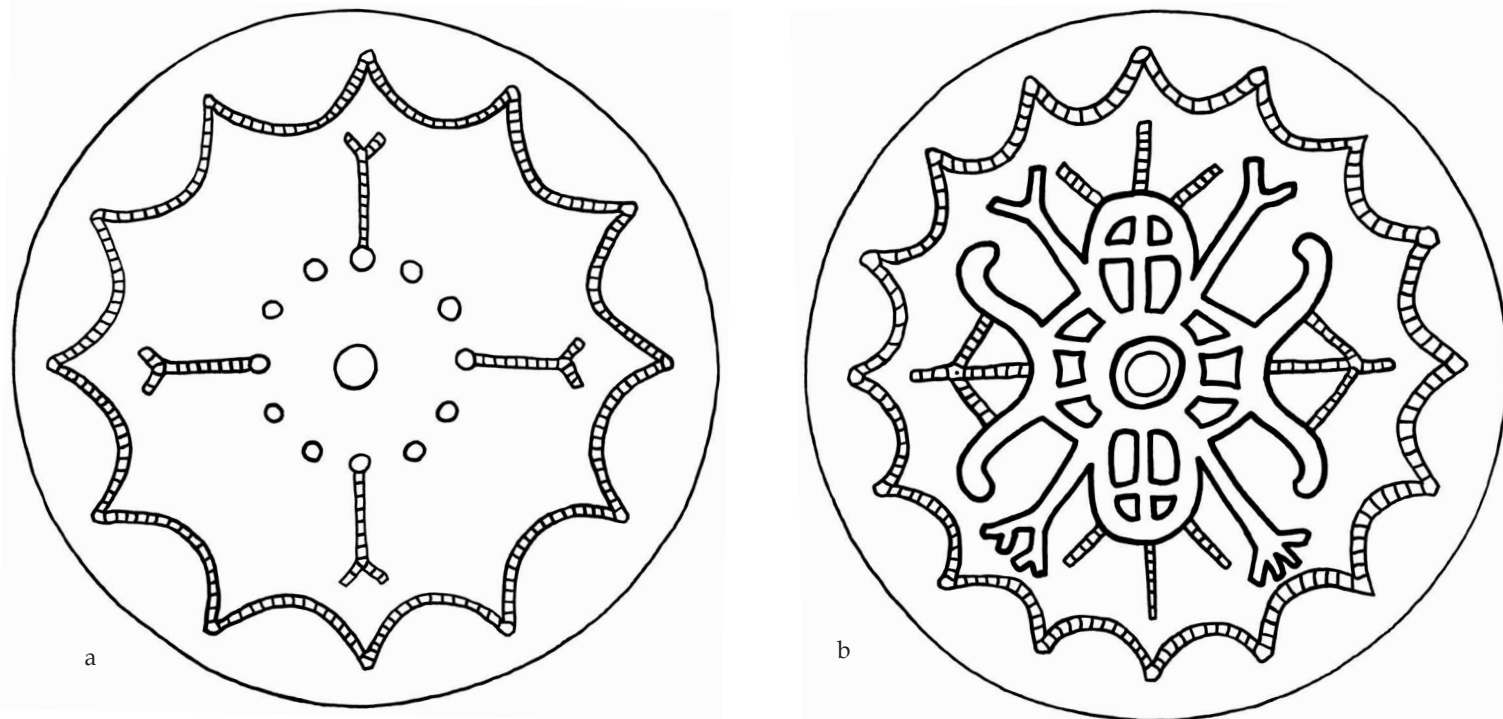
Figura 8. Recipientes coras de guaje para ofrenda y su iconografía: (a) interior del tazón con los cuatro rumbos y disco central que representa al sol (conforme a Preuss, 1998a: fig. 24.3a); (b) interior de tazón con representación del mundo y sus cuatro rumbos y diosa de la tierra y de la luna en el centro (conforme a Preuss, 1998a: fig. 24.3b).
