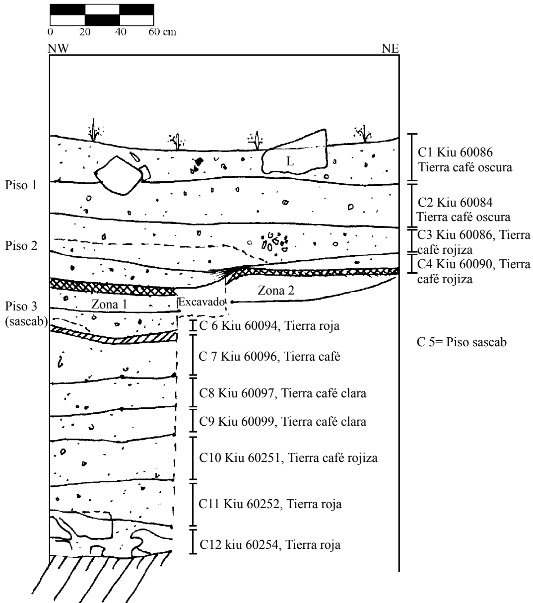
Figura 4-116. Cala 25, Cuadro B25. Perfil norte.
