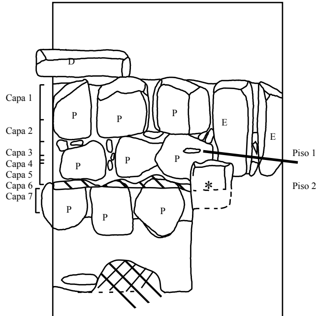
Figura 4-16. Estructura N1050E1065. Perfil este de la Unidad A'30; nótese los Pisos 1 y 2.
