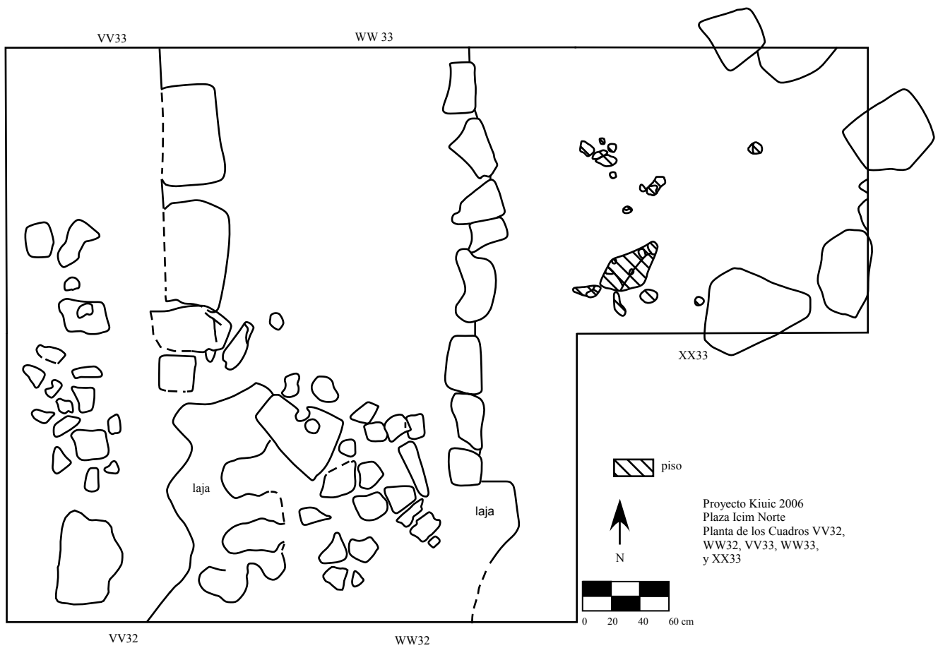
Figura 4-144. Plaza Icim Norte. Planta de las Unidades VV32/33, WW32/33 y XX33; nótese la plataforma encontrada en estas unidades.
