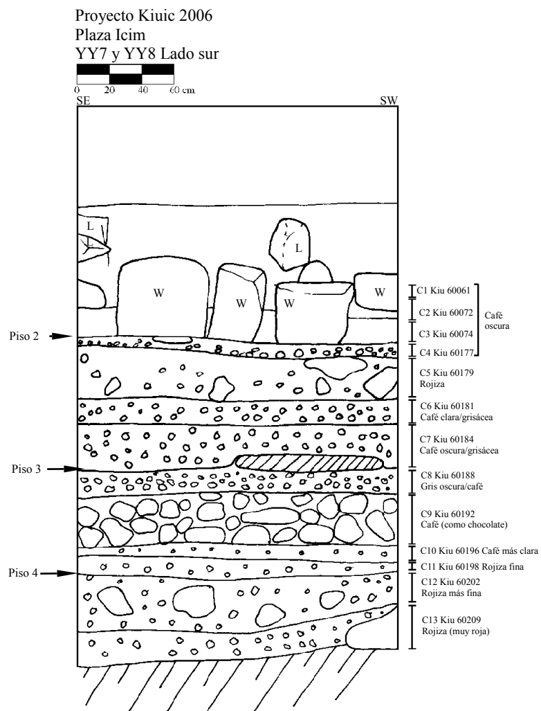
Figura 4-93. Pozo YY8. Perfil sur.
