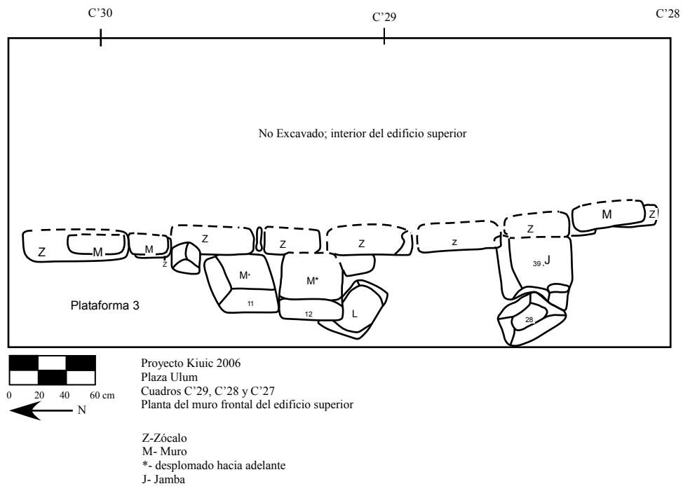
Figura 4-40. Estructura N1050E1065. Planta del muro frontal del edificio superior.
