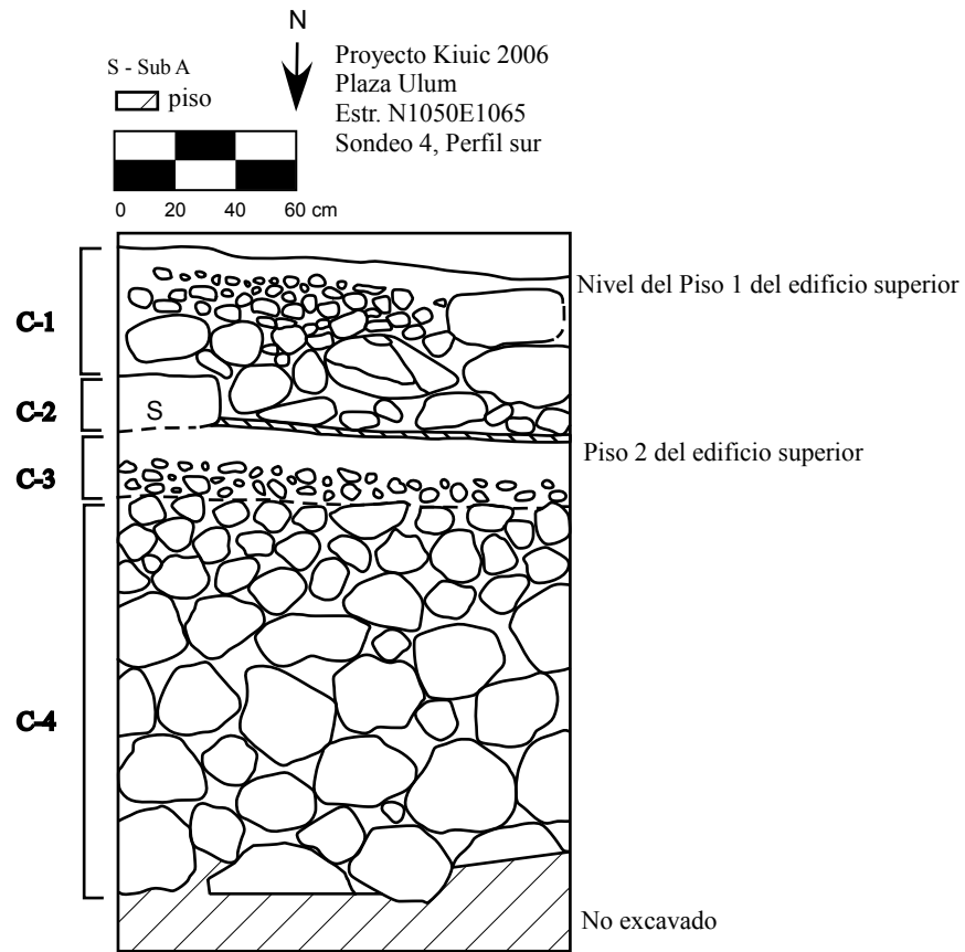
Figura 4-51. Estructura N1050E1065. Sondeo 4. Perfil sur.
