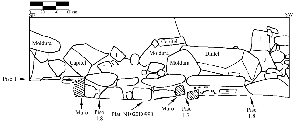
Figura 4-68. Cala 7. Perfil sur de los Cuadros ZZ7 y A7.
