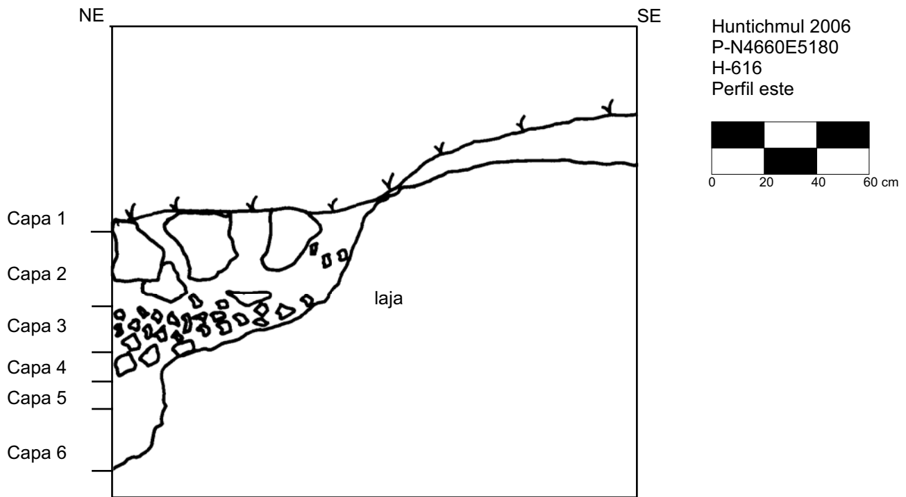
Figura 5-38. Plataforma P-N4660E5180. Unidad H-616, perfil este.
