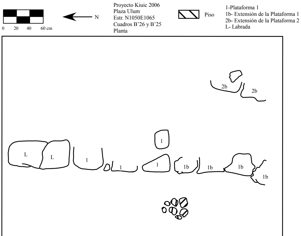
Figura 4-19. Estructura N1050E1065. Planta de las Plataformas 1 y 2, lado sur.
