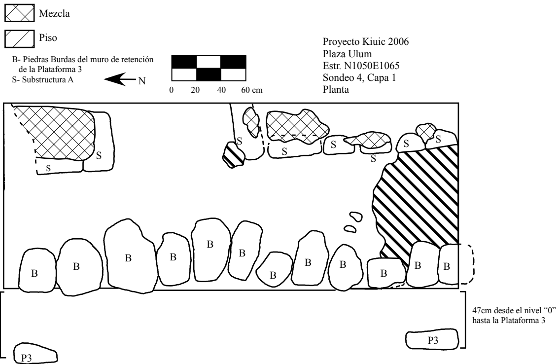
Figura 4-45. Estructura N1050E1065. Sondeo 4, Capa 1. Planta de las piedras alineadas.
