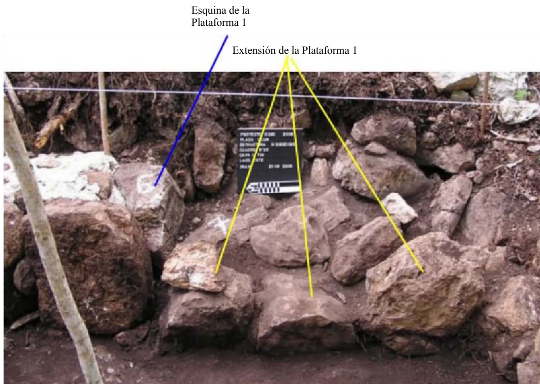
Figura 4-22. Estructura N1050E1065. Esquina sur de la Plataforma 1.
