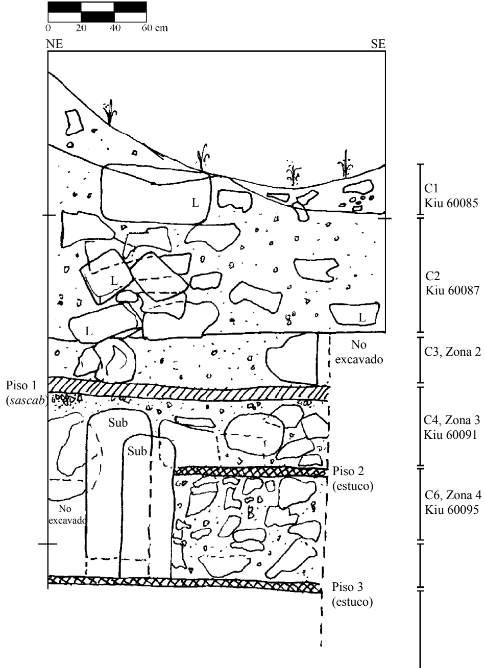
Figura 4-137. Cala 25, Cuadro F25. Perfil este.
