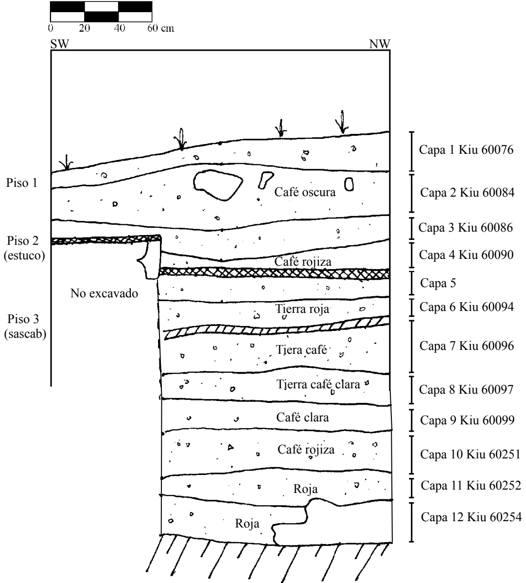
Figura 4-115. Cala 25, Cuadro B25. Perfil oeste.
