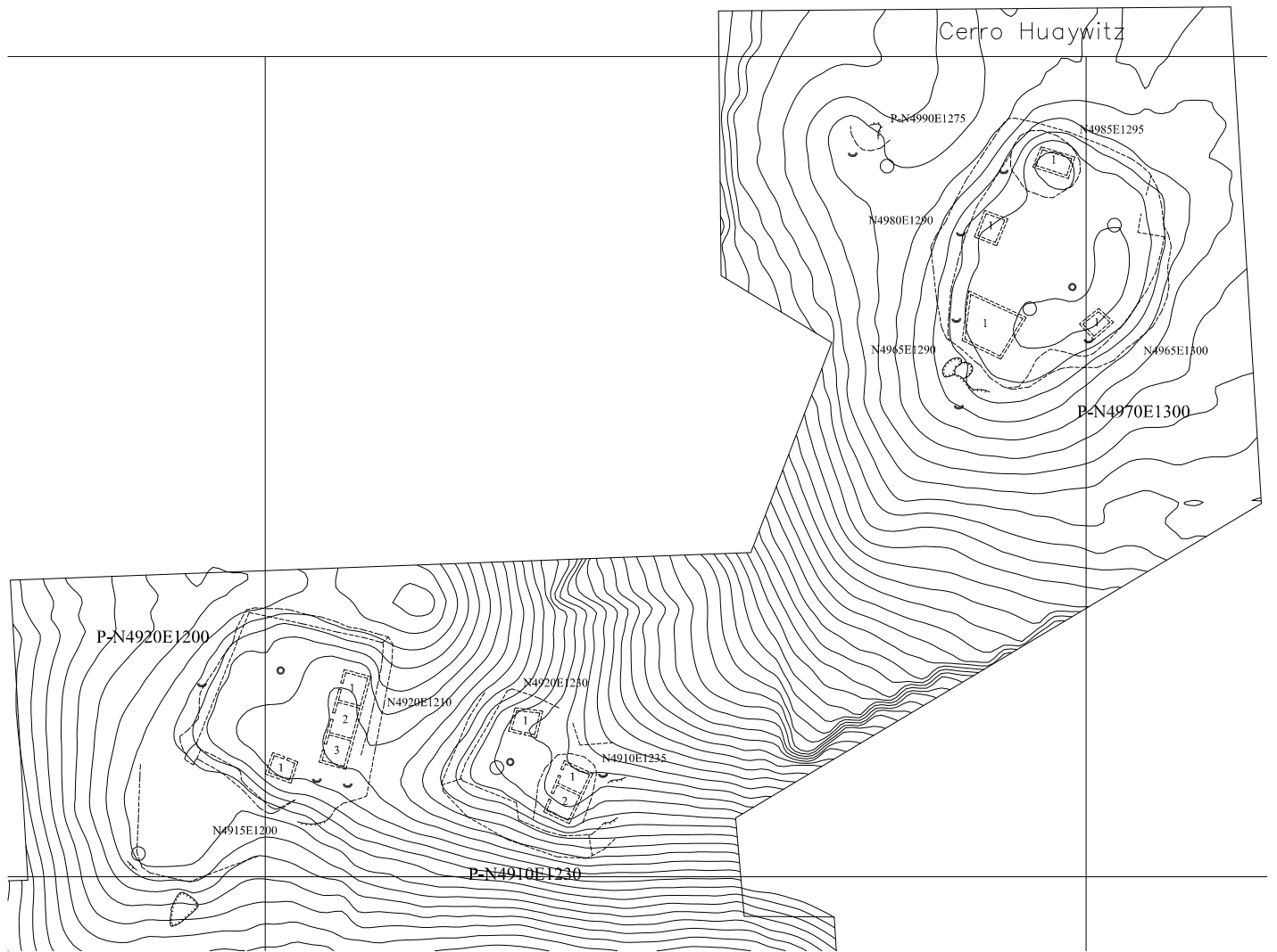
Figura 3-19. Las Plataformas P-N4920E1200, P-N4910E1230 y P-N4970E1300 (la cuadrícula mide 100 m).
