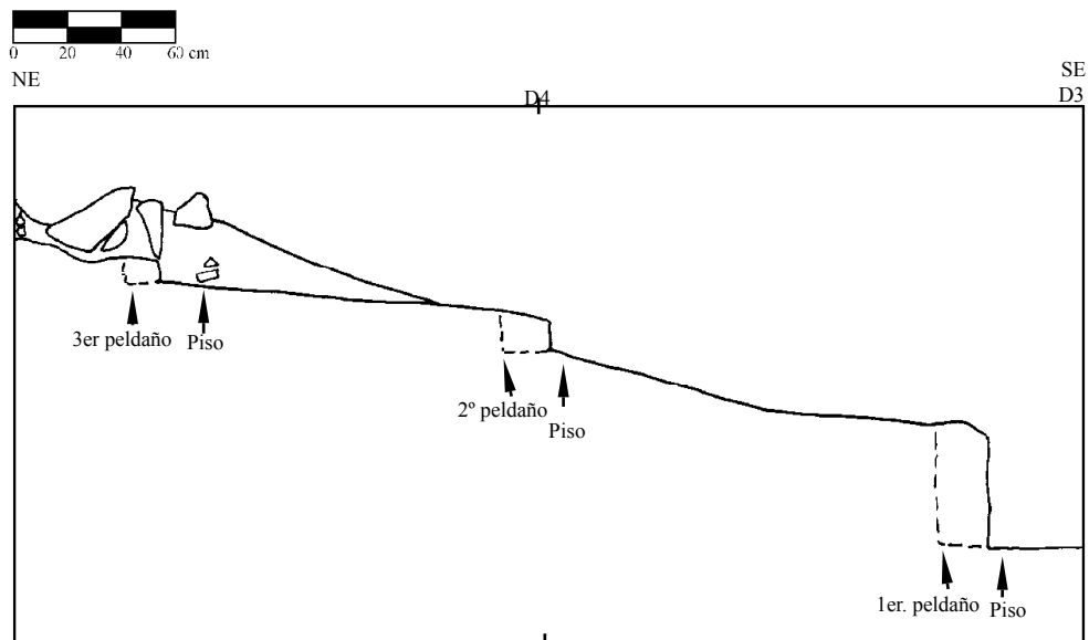
Figura 4-57. Cala D. Perfil este del acceso a la Plaza Icim.
