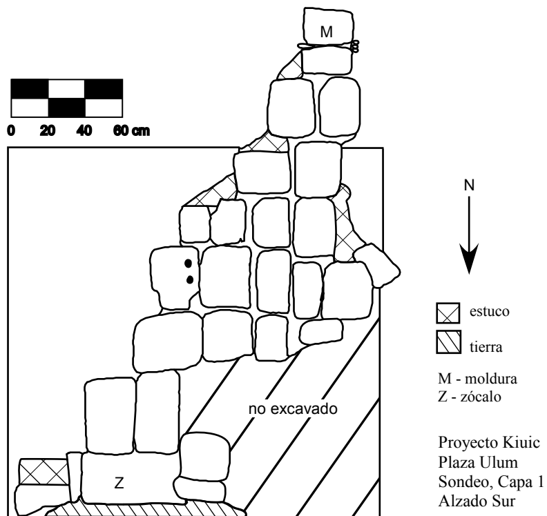
Figura 4-6. Estructura N1050E1065. Alzado mostrando la moldura hallada in situ en el muro norte del edificio superior.
