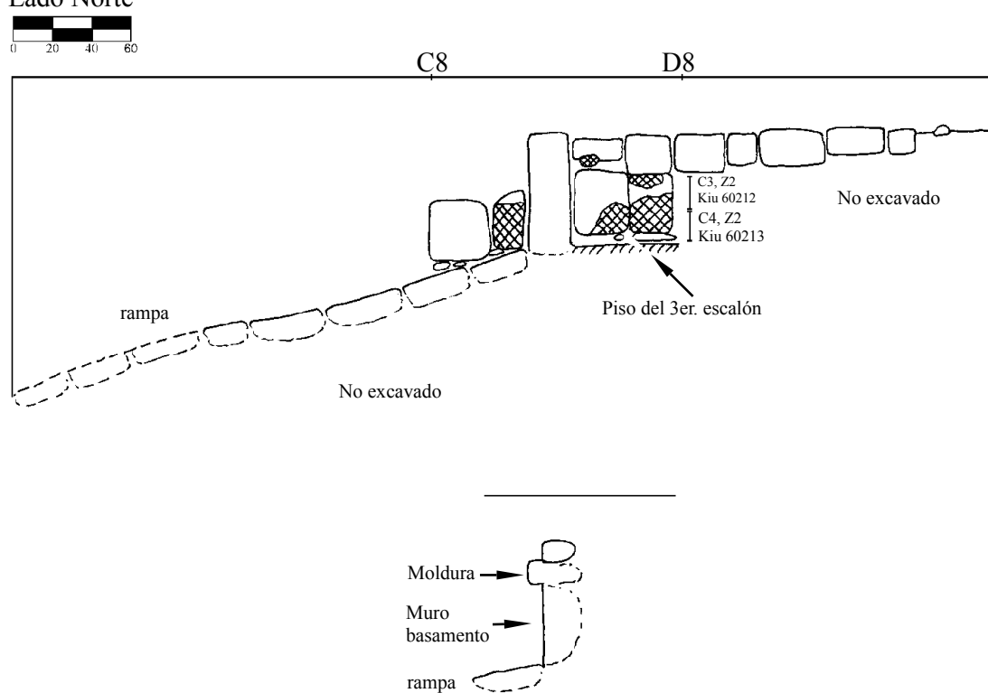
Figura 4-72. Cuadro C9. Alzado del muro sur del basamento con moldura y la rampa; abajo detalle del perfil del basamento y su unión con la rampa.
