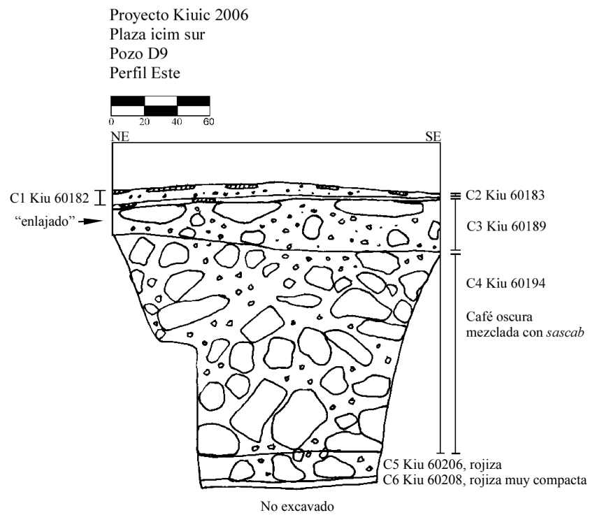
Figura 4-79. Pozo D9. Perfil este.
