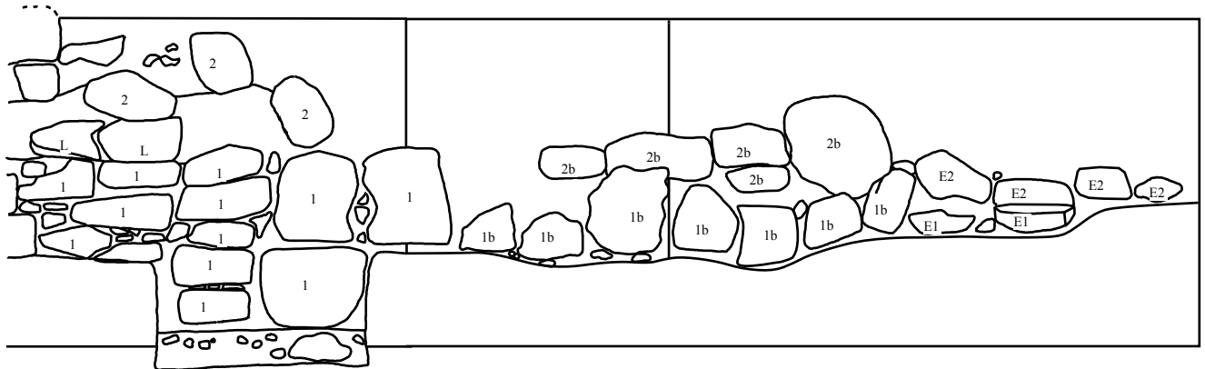
Figura 4-25. Estructura N1050E1065. Alzado este de las Plataformas 1 y 2, lado sur.
