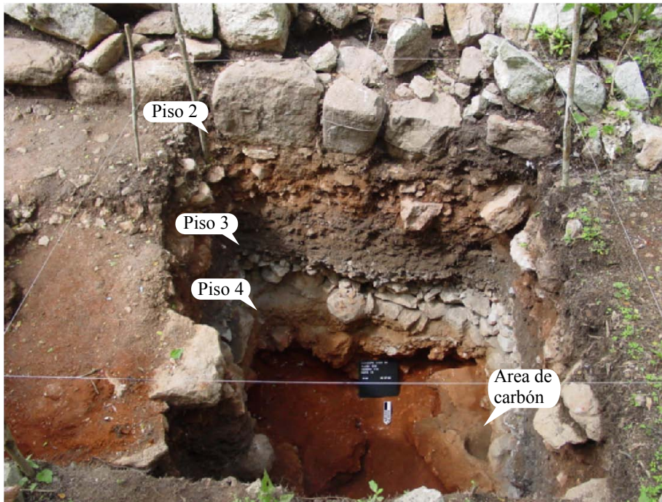
Figura 4-92. Pozo YY8. Lado sur.
