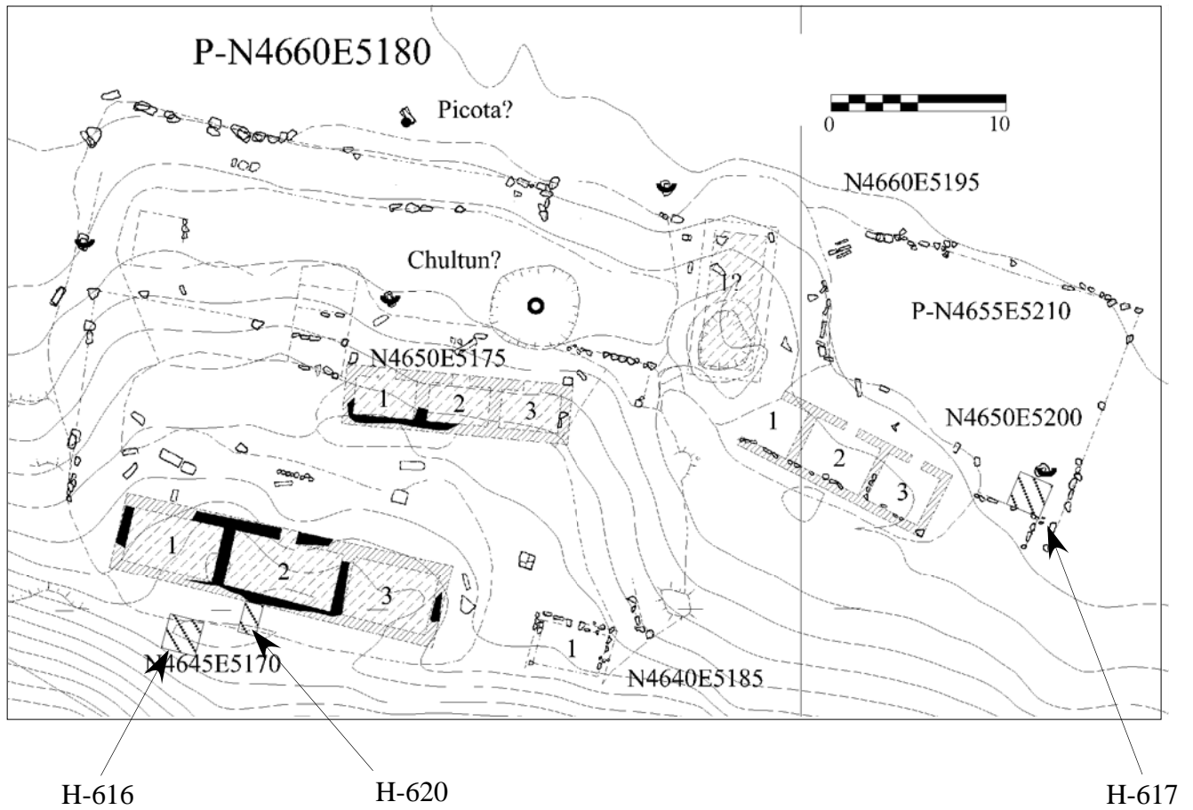
Figura 5-34. La Plataforma P-N4660E5180 mostrando las unidades excavadas.
