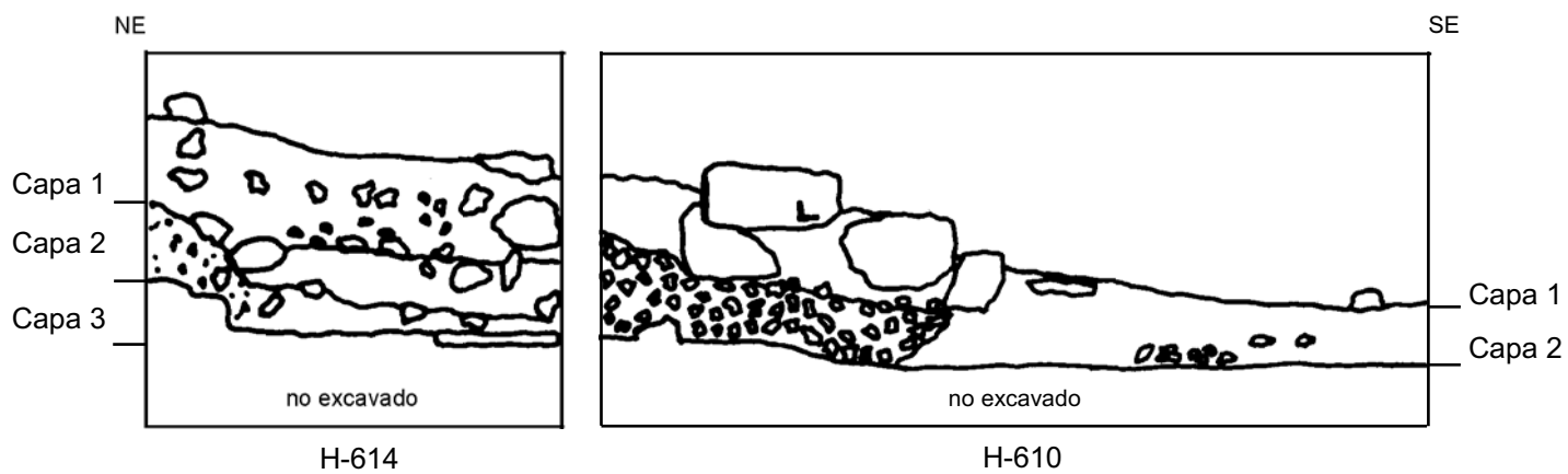
Figura 5-7. Plataforma P-N4940E5260. Unidades H-610 y H-614, perfil este.
