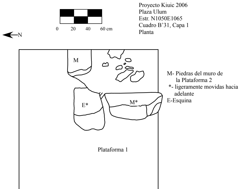
Figura 4-29. Estructura N1050E1065. Planta de la esquina NW de la extensión al lado norte de la Plataforma 2.
