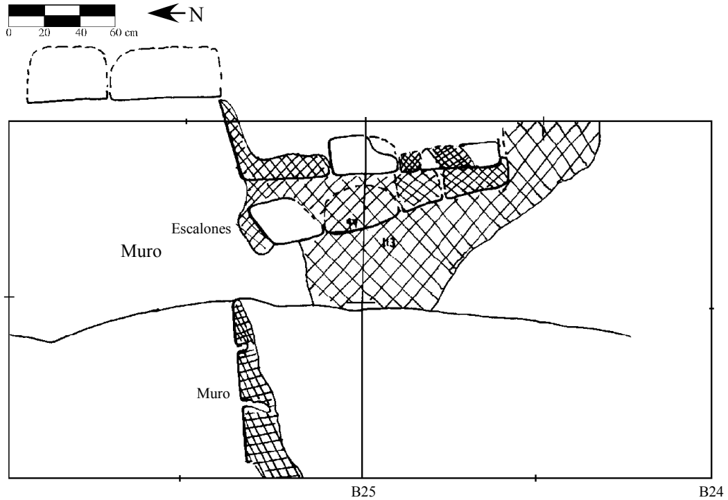
Figura 4-100. Cala B. Planta de los escalones y la plataforma en el lado este y el muro en el lado oeste.
