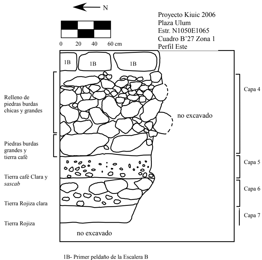
Figura 4-12. Estructura N1050E1065. Detalle del relleno constructivo de las Escaleras A y B, donde la parte inferior de la Escalera B fue desmantelada para construir la Escalera A.
