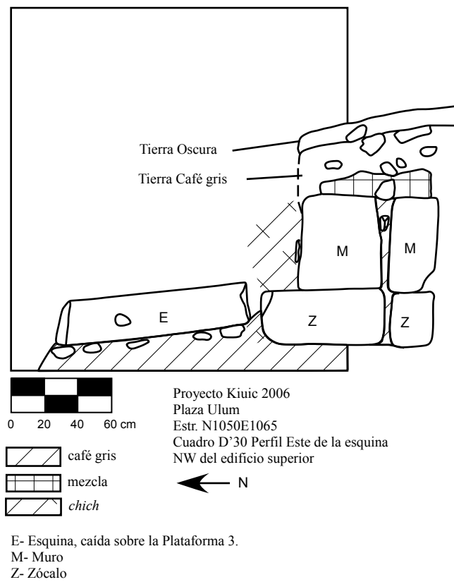
Figura 4-41. Estructura N1050E1065. Alzado de la esquina NW del edificio superior desplomada.
