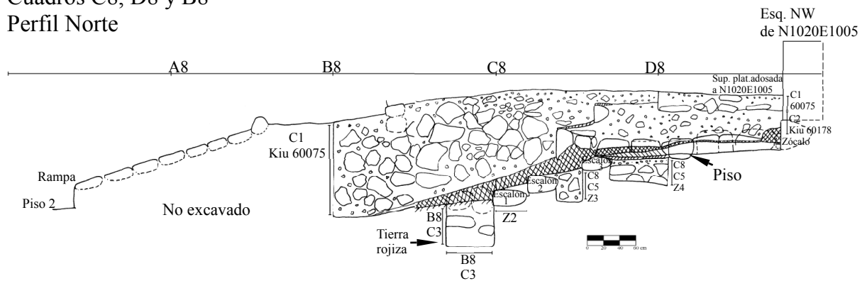
Figura 4-83. Cala 8. Perfil norte.
