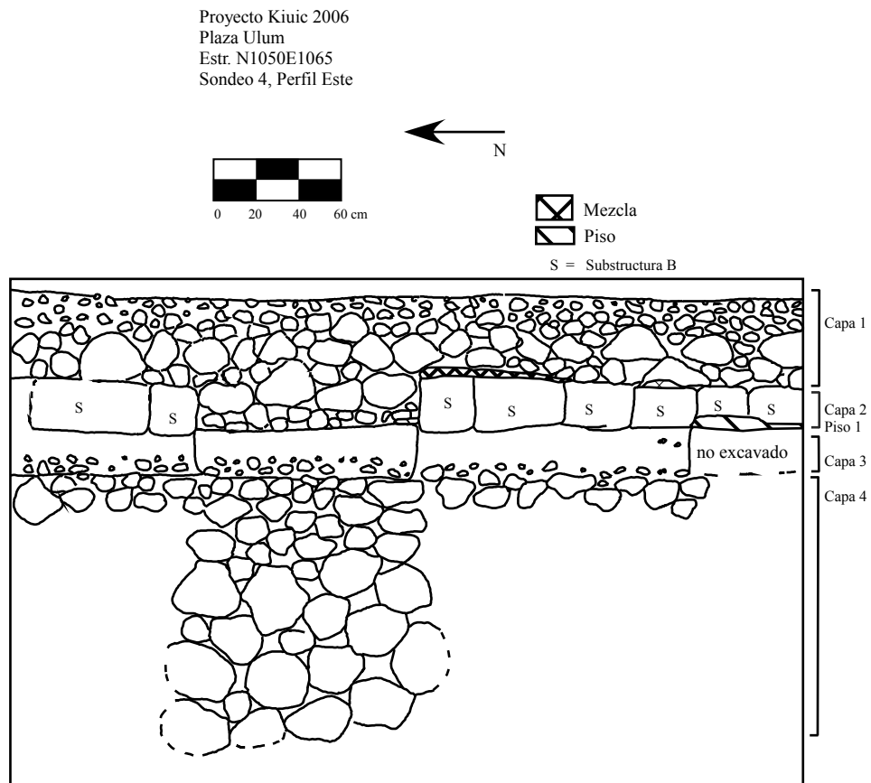
Figura 4-50. Estructura N1050E1065. Sondeo 4. Perfil este.
