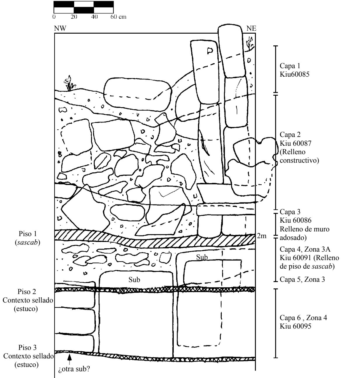
Figura 4-136. Cala 25, Cuadro F25. Perfil norte.
