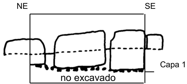
Figura 5-30. El Grupo Chanchich. Unidad H-621, perfil este.
