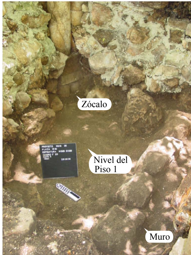
Figura 4-128. Cala 25, Cuadro F25. Detalle del zócalo del Cuarto 4 de la Estr. N1065E1025 y el muro hallado en el lado sur de la unidad.
