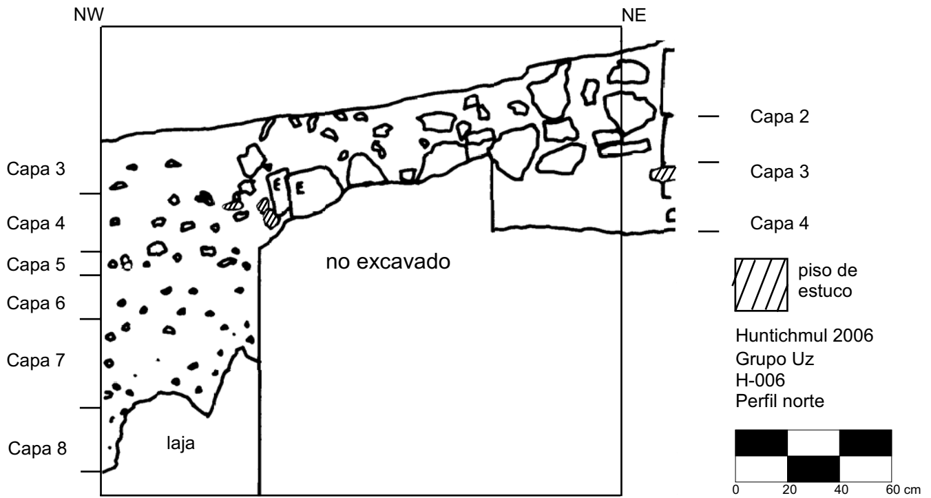
Figura 5-46. El Grupo Uz. Unidad H-006, perfil norte.
