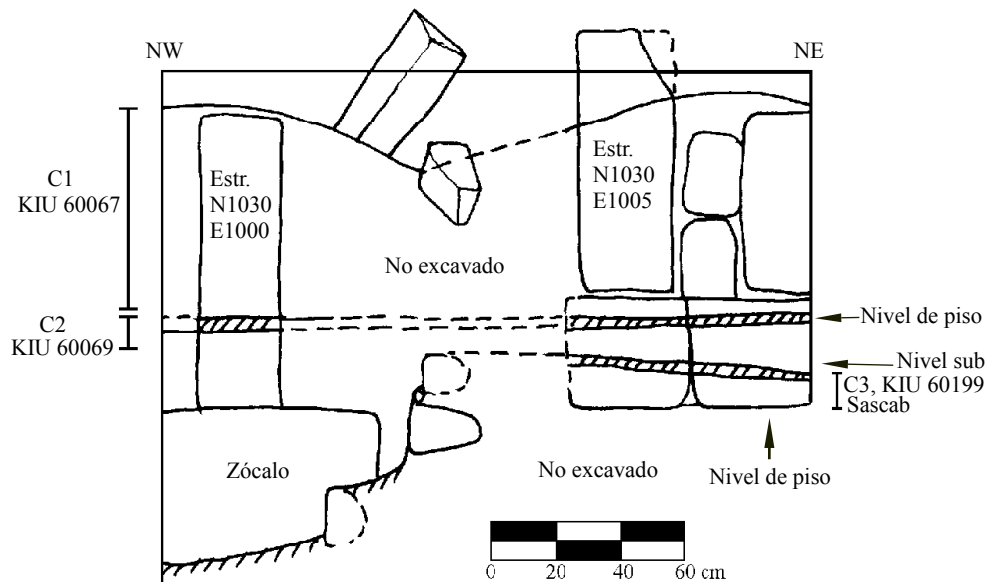
Figura 4-87. Cuadro C10. Alzado, lado norte.
