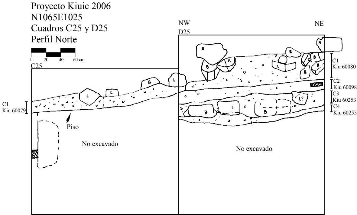
Figura 4-120. Cala 25, Cuadros C25 y D25. Perfil norte.
