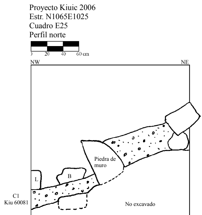
Figura 4-125. Cala 25, Cuadro E25. Perfil norte.
