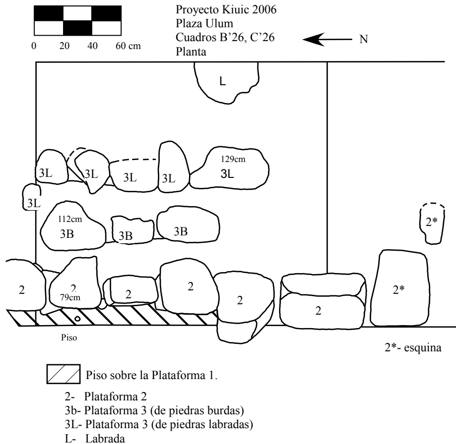
Figura 4-32. Estructura N1050E1065. Planta del lado sur de la Plataforma 2.
