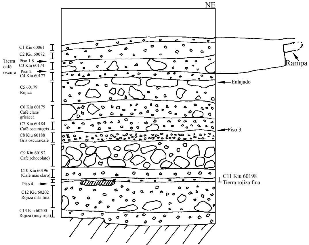
Figura 4-96. Pozo YY8. Perfil norte.
