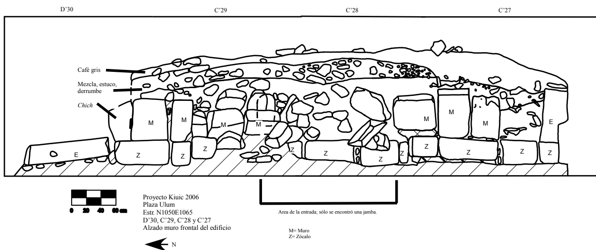
Figura 4-39. Estructura N1050E1065. Alzado del muro frontal (oeste) del edificio superior.
