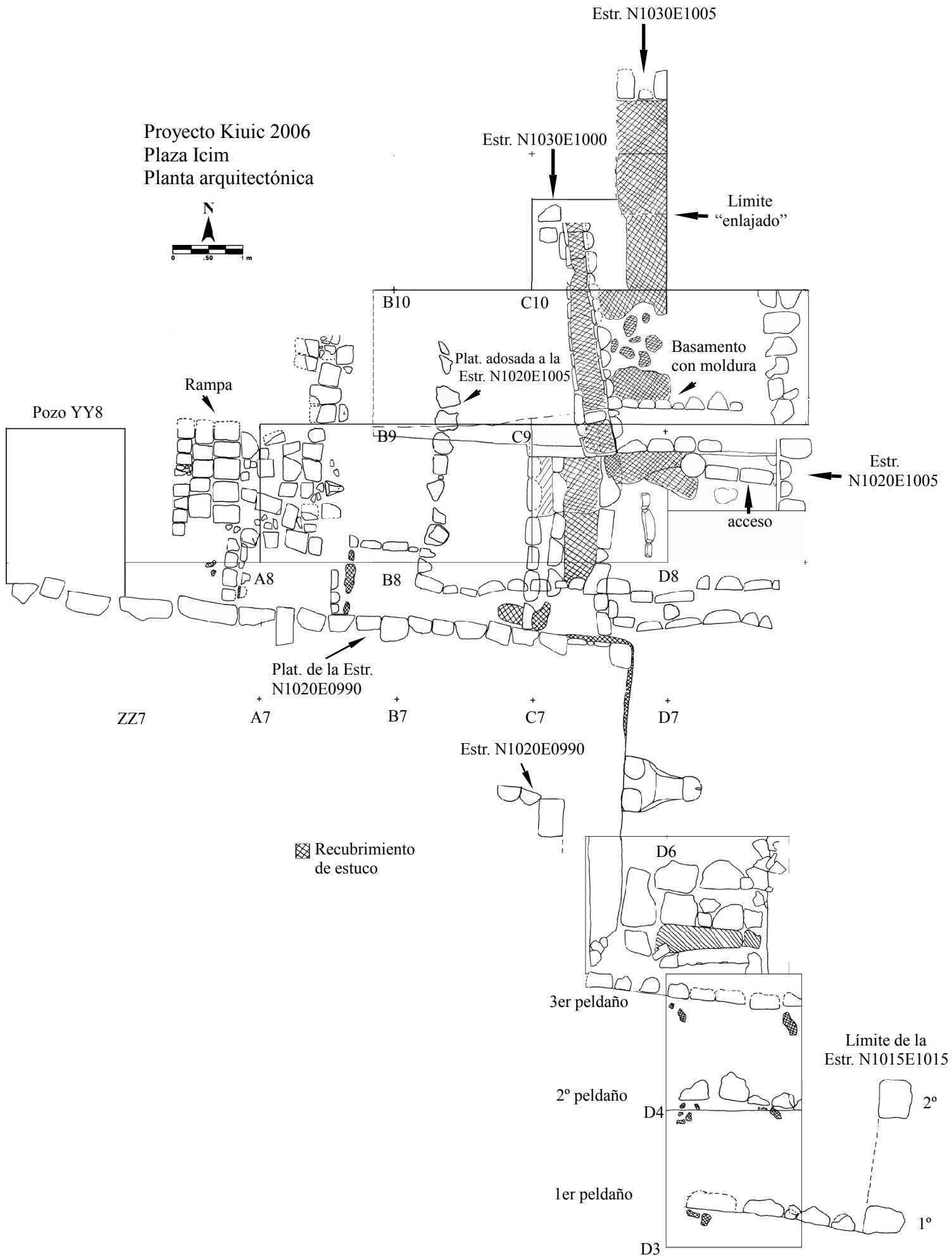
Figura 4-55. Planta arquitectónica del sector sureste de la Plaza Icim.
