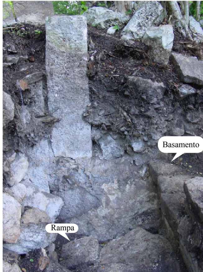
Figura 4-88. Cuadro C10. Detalle de la unión de la rampa con el basamento con moldura.
