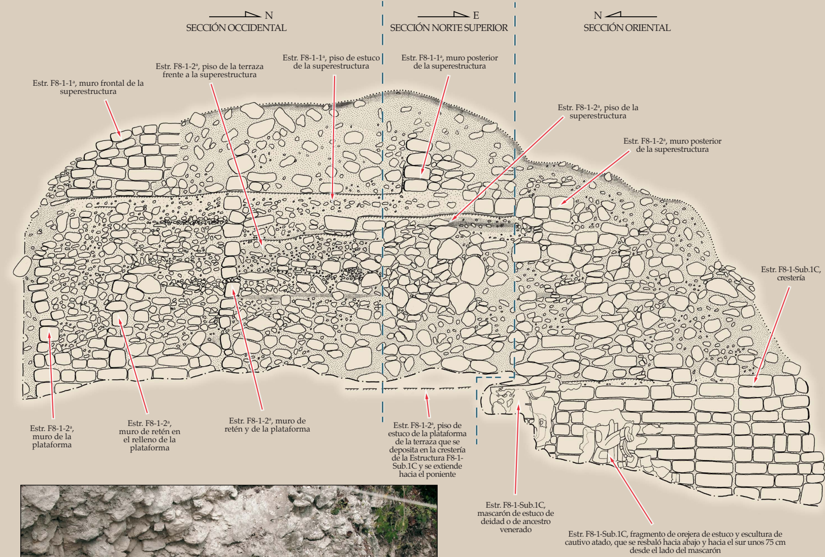
Figura 2.4. Perfil de excavación de la zanja de saqueo ya limpia, lado sur de la Estructura F8-1, con elementos arquitectónicos de la Estructura F8-1-Sub.1C, F8-1-1ª y F8-1-2ª. En el dibujo y en la fotografía de la izquierda pueden verse restos de estuco modelado de la crestería de la Estructura Sub.1C, el llamado "Templo del Sol Nocturno." El mascarón de estuco de Chahk que aparece en el extremo derecho del dibujo y en las vistas adyacentes, proviene de la fachada sur de Sub.1C (ver Capítulo 5). Dibujo: Nicholas Carter; fotos: Arturo Godoy; fotogrametría: Katie Simon, CAST.
