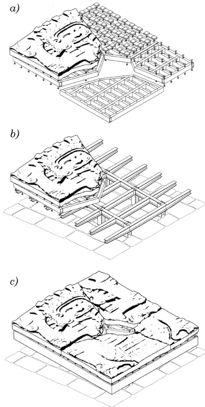
FIGURA 156. a) Soportes individuales. Sistema de pernos roscados y apoyos deformables; b) soportes individuales sobre base fija; c) vista de los cuatro fragmentos sobre la base museográfica definitiva (CFE).
